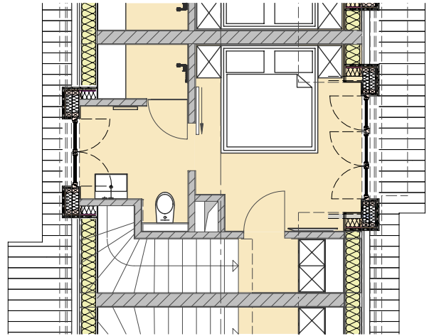
Obergeschoss
